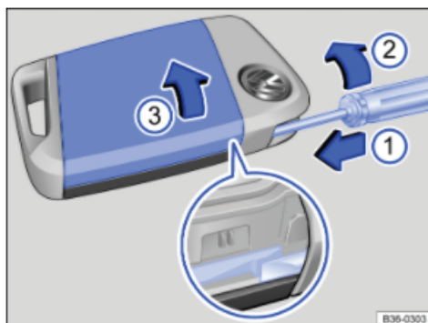
איור 1. מפתח הרכב: פתיחת כיסוי תא סוללה
