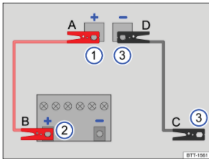
איור 2. תרשים לחיבור כבלי התנעה ברכב המסייע (מצבר 12 וולט בתא המטען)
